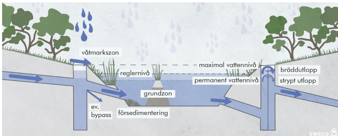
Figur 3 Tvärsektion utformning dagvattendamm.
